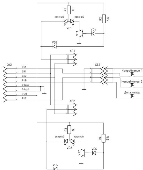
Схема электрическая принципиальная ПДУ
